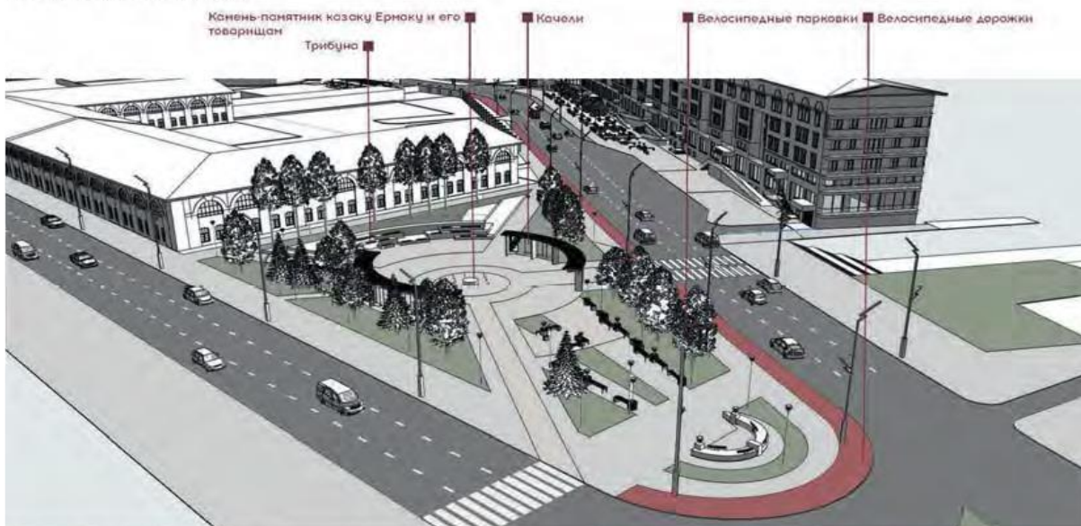
ПЕРСПЕКТИВНЫЙ ВИД НА ВЕЛОПАРКИНГ
