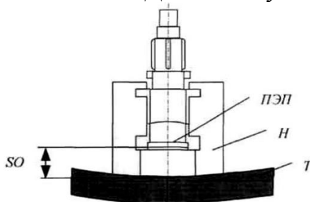
Рисунок 2.1 - Схема установки пьезоэлектрического преобразователя в упругом носителе внутритрубного дефектоскопа ПЭП - пьезоэлектрический преобразователь; Т - трубопровод; SO- значение отступа; Н- носитель датчиков ПЭП
