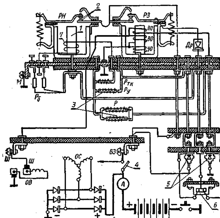
Рис. 3.1. Схема генераторной установки переменного тока:
