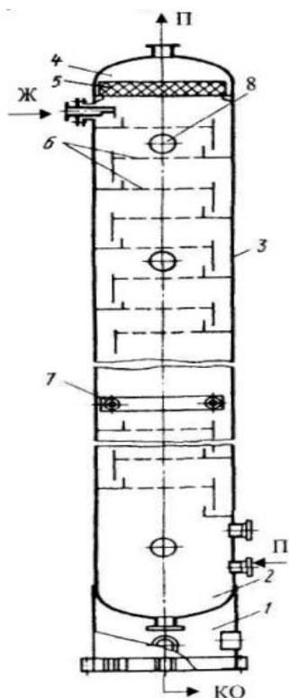
1 – опорная обечайка; 2,4 – днища; 3 – корпус; 5 – отбойное устройство; 6 – тарелки; 7 – устройство ввода сырья; 8 – люки для обслуживания Рисунок 5.1 – Эскиз ректификационной колонны
