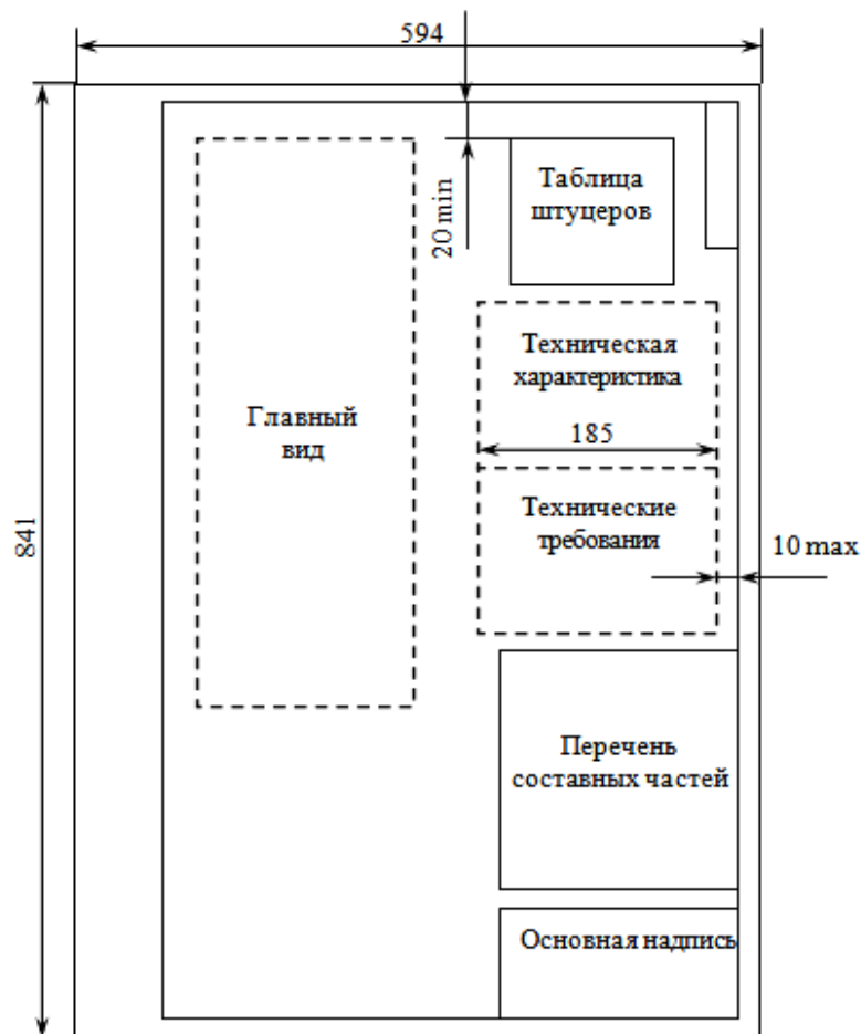
Рисунок 6.3 - Расположение основных элементов (вертикальный лист)
