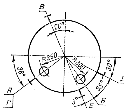
Рисунок 6.1. Схема расположения штуцеров
