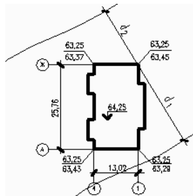
Рисунок 3 - Определение проектных и фактических отметок
