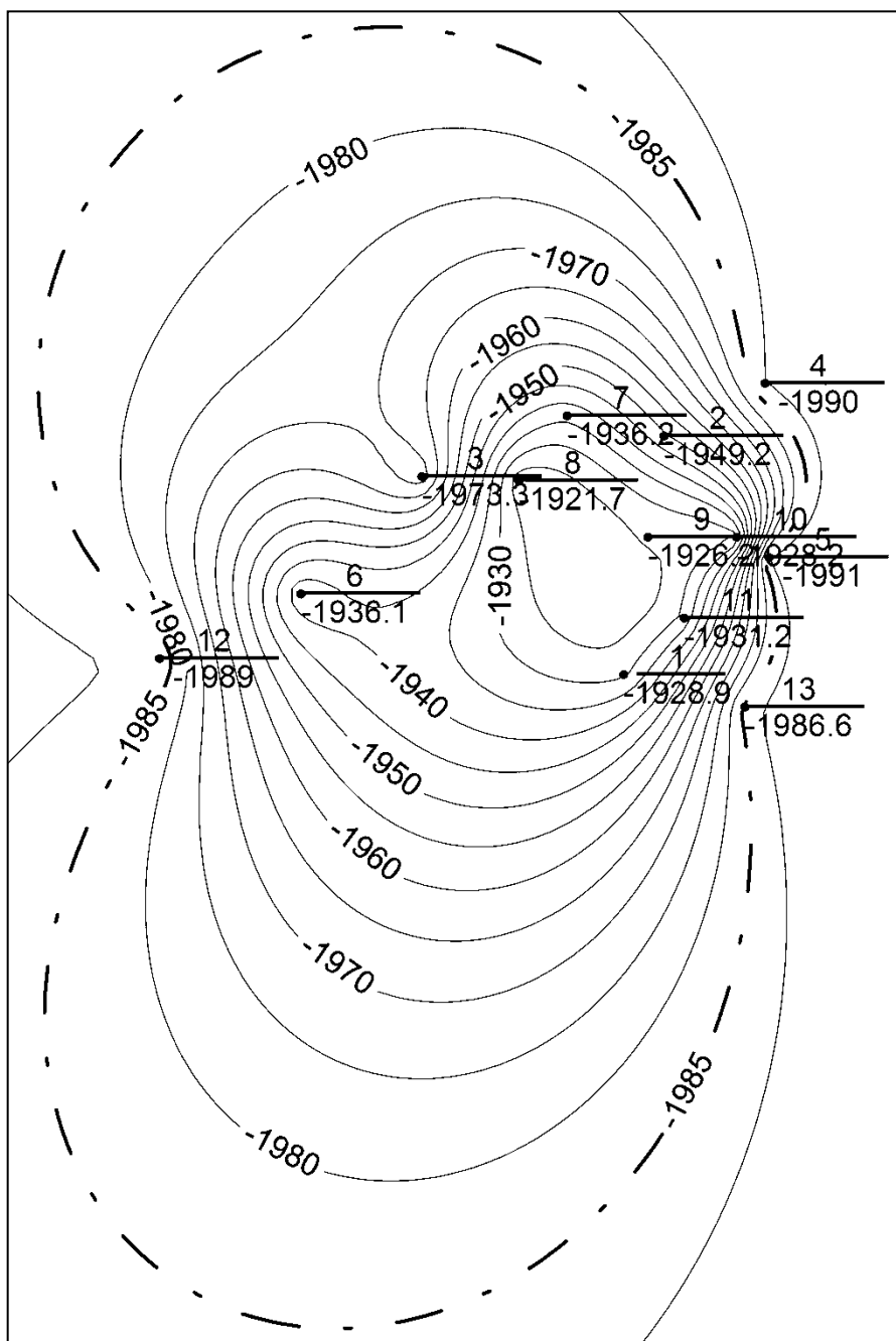
Рисунок 3 - Структурная карта по кровле продуктивного пласта
