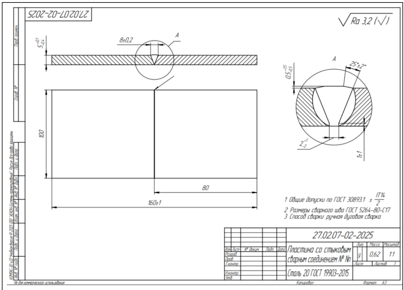
Рисунок 1 – Чертеж пластины
