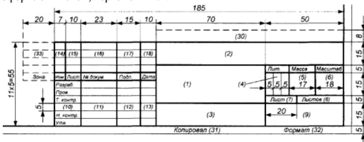
Рисунок 1 – Основная надпись Форма 1
