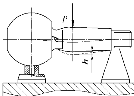
Рисунок 1 - Проверка прочности шарового пальца
