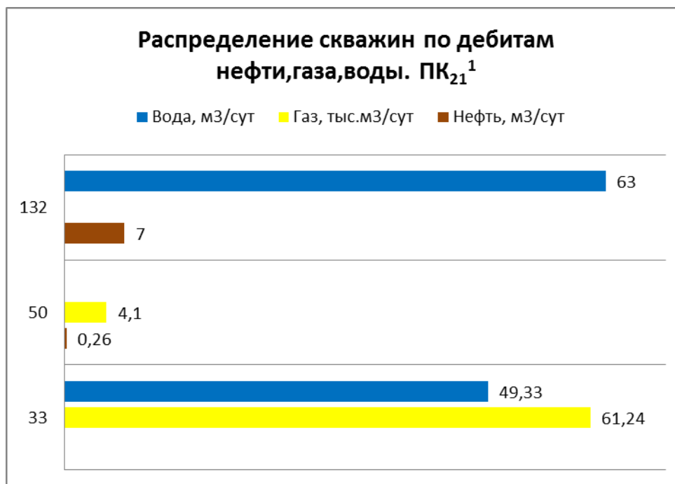
Рисунок 2.1 – Распределение скважин по дебитам нефти, газа, воды. Пласт ПК 21 1
