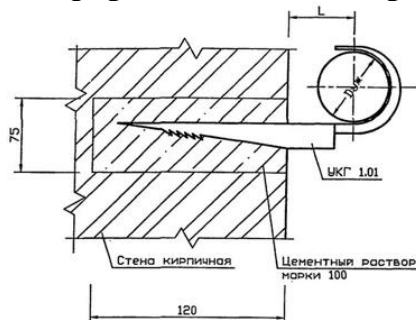
Рисунок 2 – Крепление газопровода к стене
