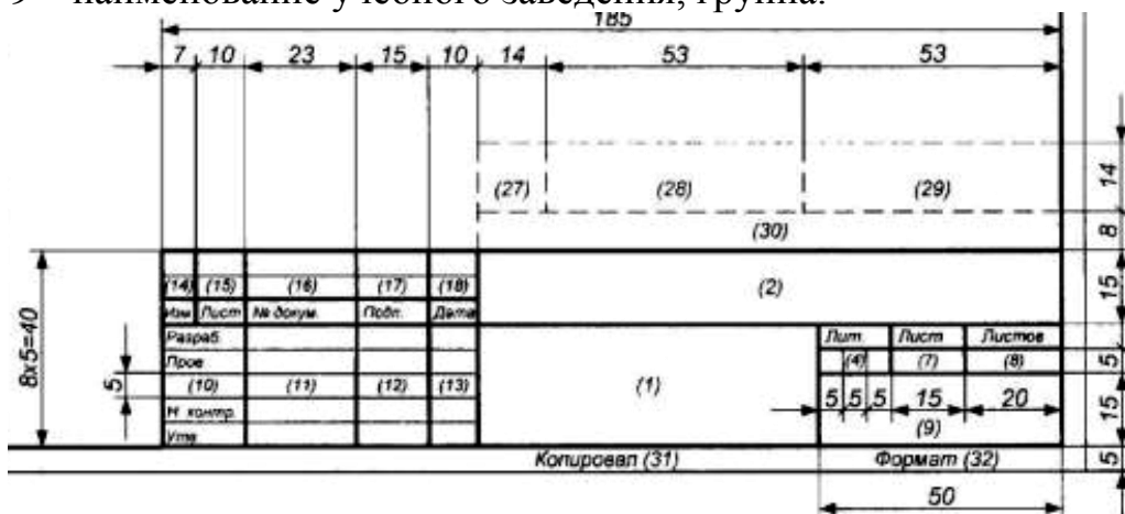
Рисунок 2 - Основная надпись Форма 2
