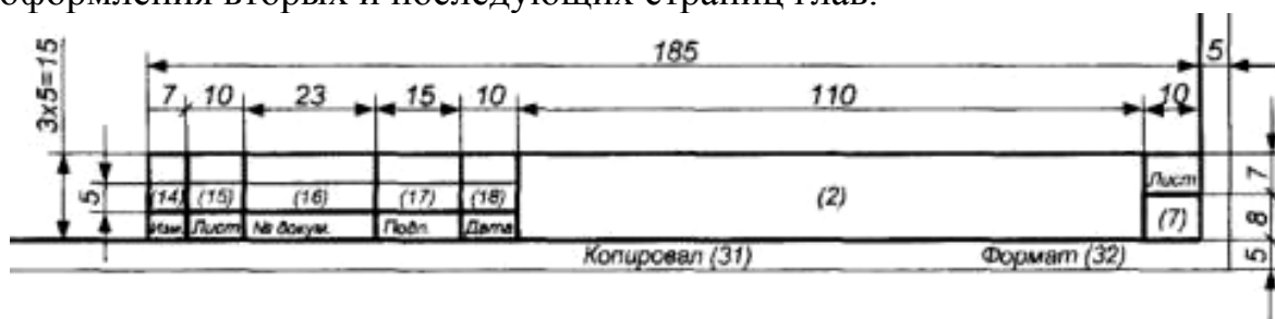
Рисунок 3 - Основная надпись Форма 2,а
