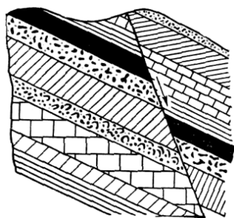
Рис. 14. Сброс
