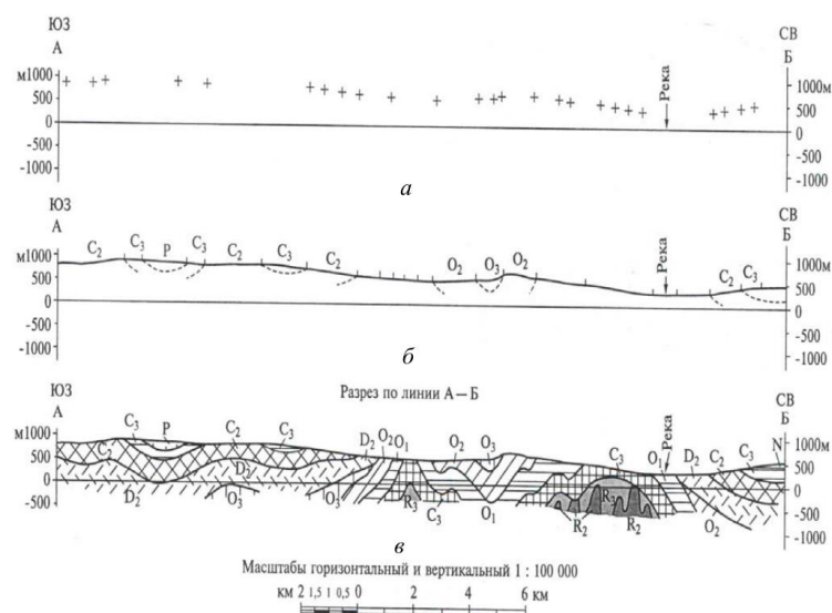
Рис. 21. Этапы построения геологического разреза
