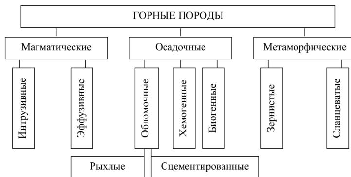
Рис. 4. Классификация горных пород по происхождению и условию залегания
