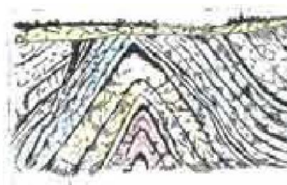
Рис. 11. Антиклиналиальная складка
