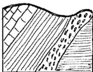
Рис. 7. Моноклиналь
