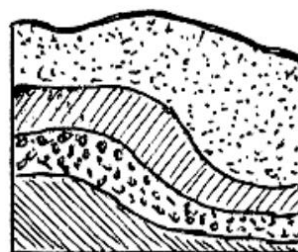
Рис. 8. Флексура
