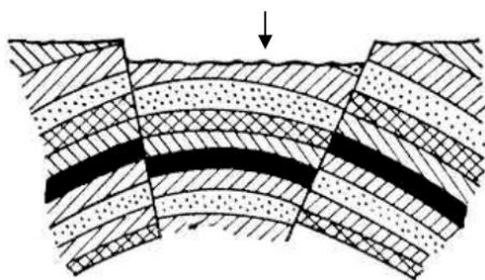
Рис. 16. Сброс
