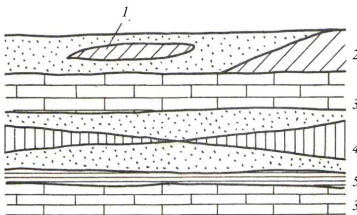
Рис. 5. Первичные формы залегания осадочных пород: 1 – линза; 2 – выклинивание; 3 – слой; 4 – пережим; 5 – прослой.
