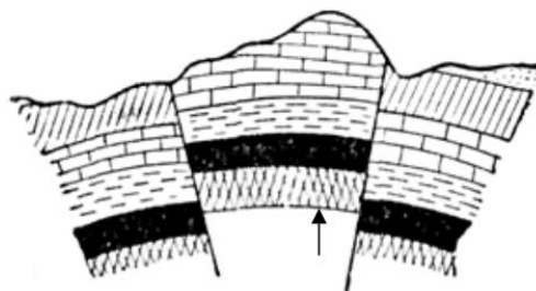
Рис. 17. Взброс
