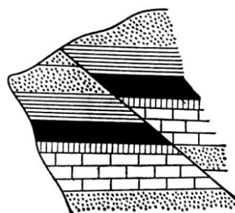
Рис. 15. Взброс
